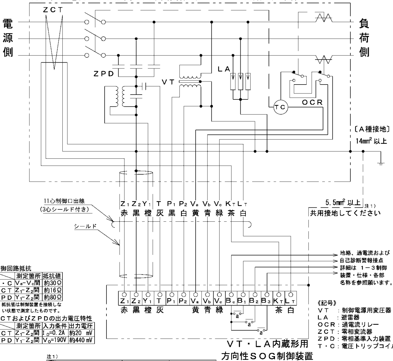
方向性過電流ロック形高圧気中開閉器（VT・LA内蔵形）本体
