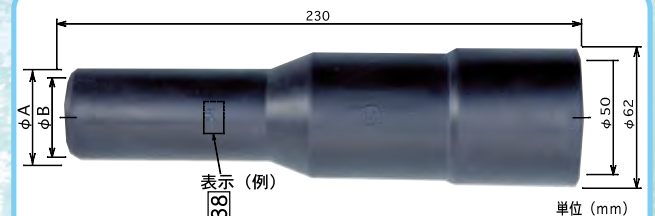
端子カバー
