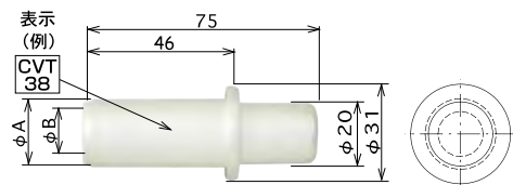
圧縮端子
