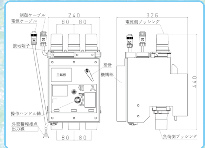
取付金具（自立用）外形図
