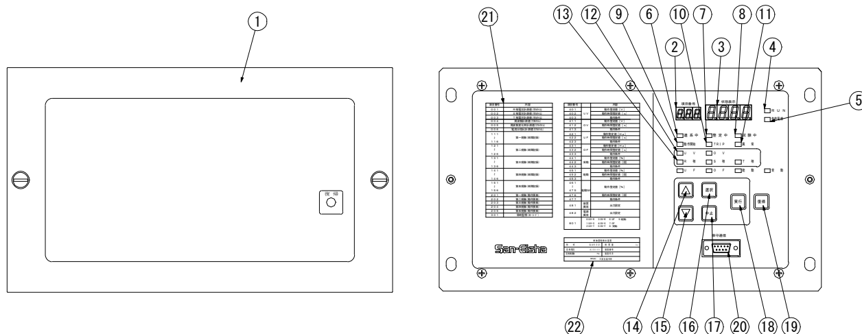
図 III-1 装置（正面）説明一覧表
