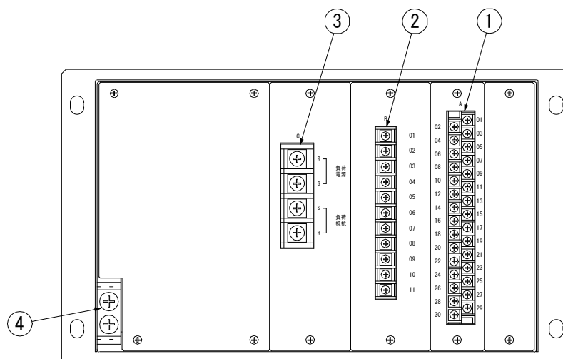
図 III-2 装置（背面）説明一覧表
