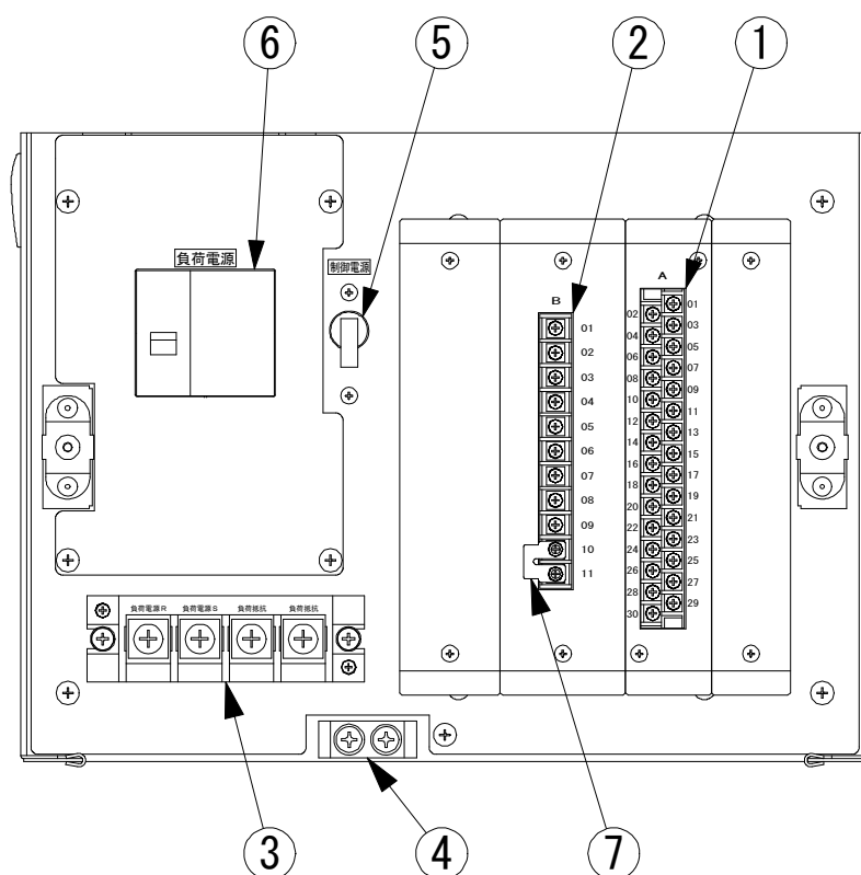
図 III-3 装置（下部）
