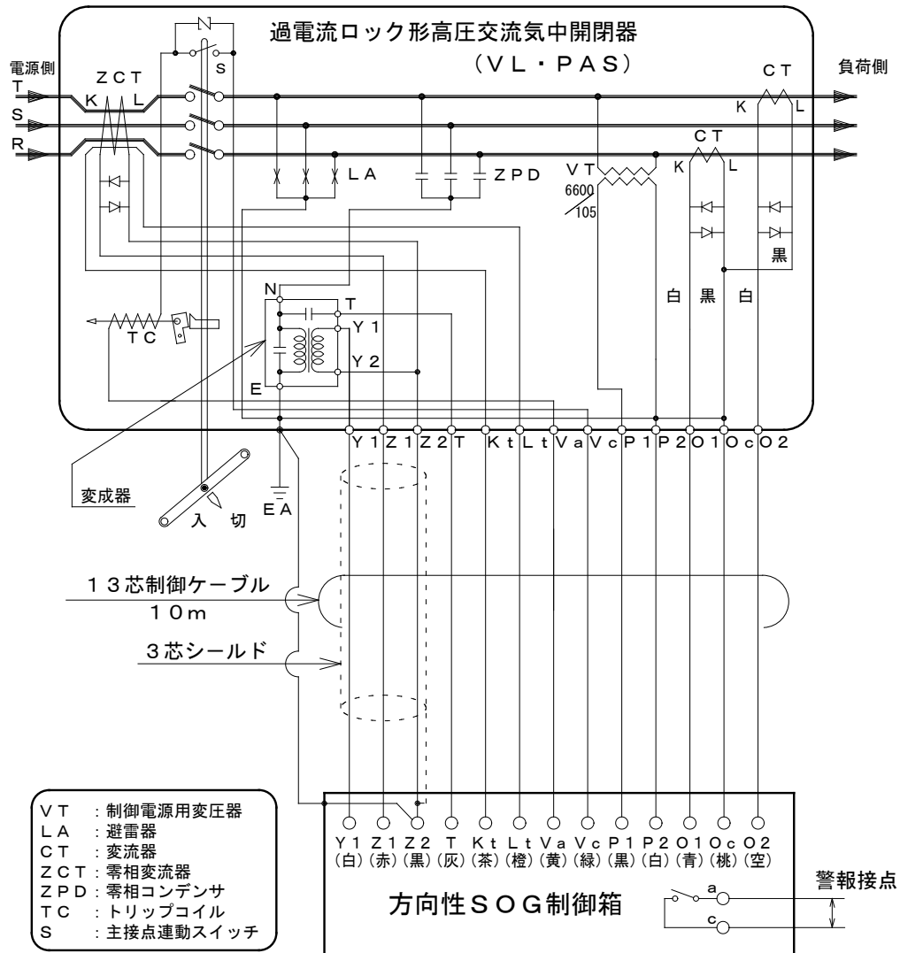
図－9 端子接続詳細銘板
