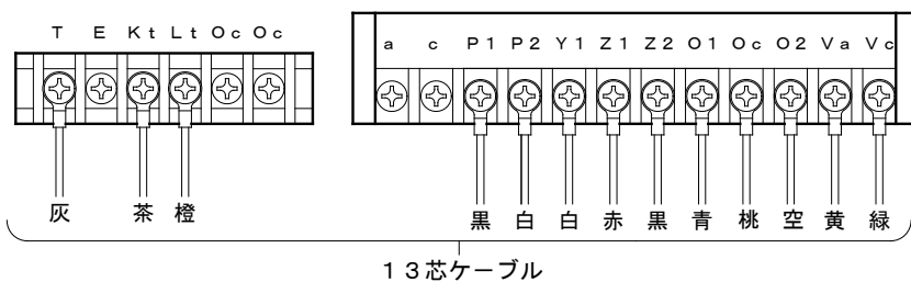
端子接続詳細図
