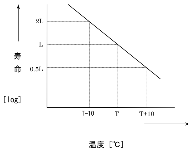
図 15. アレニウスの法則
