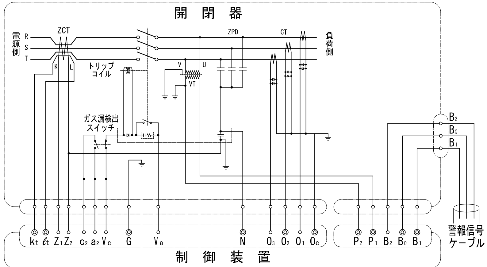
図-5 結線図
