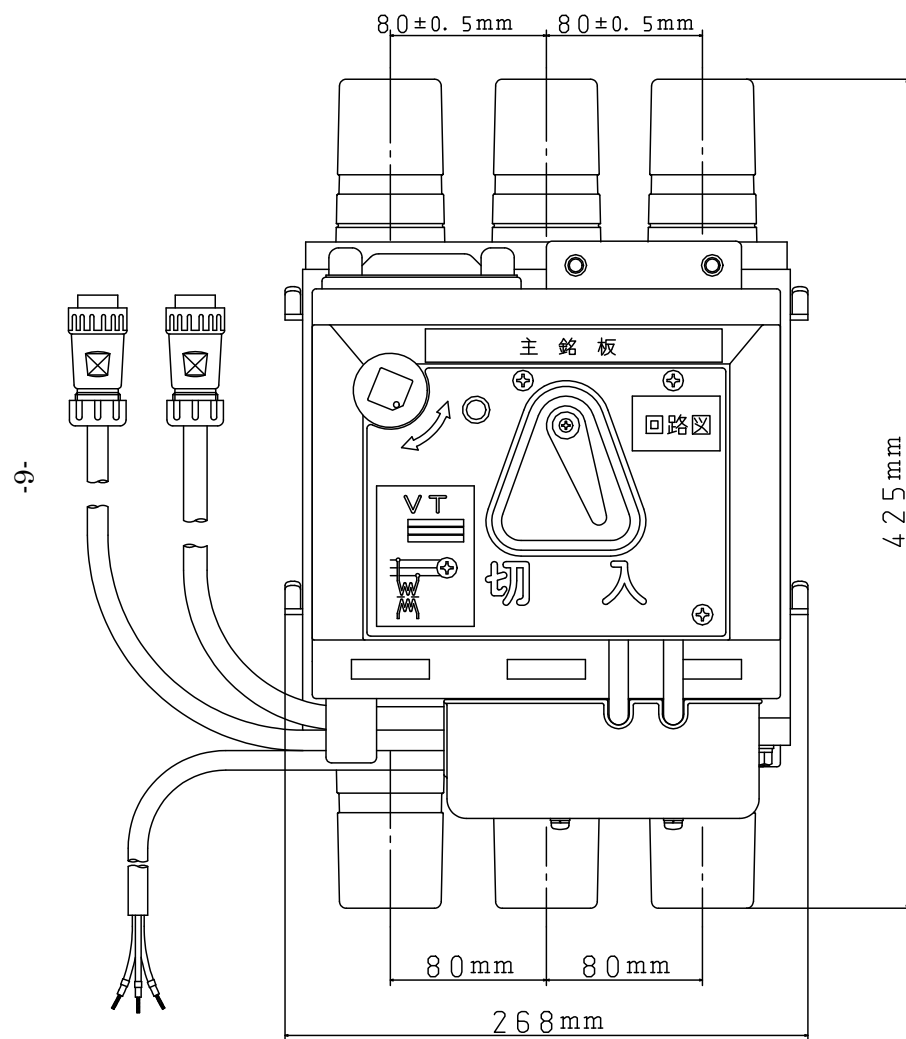
図-1 開閉器外観図（形式 SH304）
