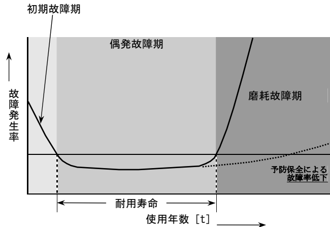
図 13. 使用年数と故障率の関係
