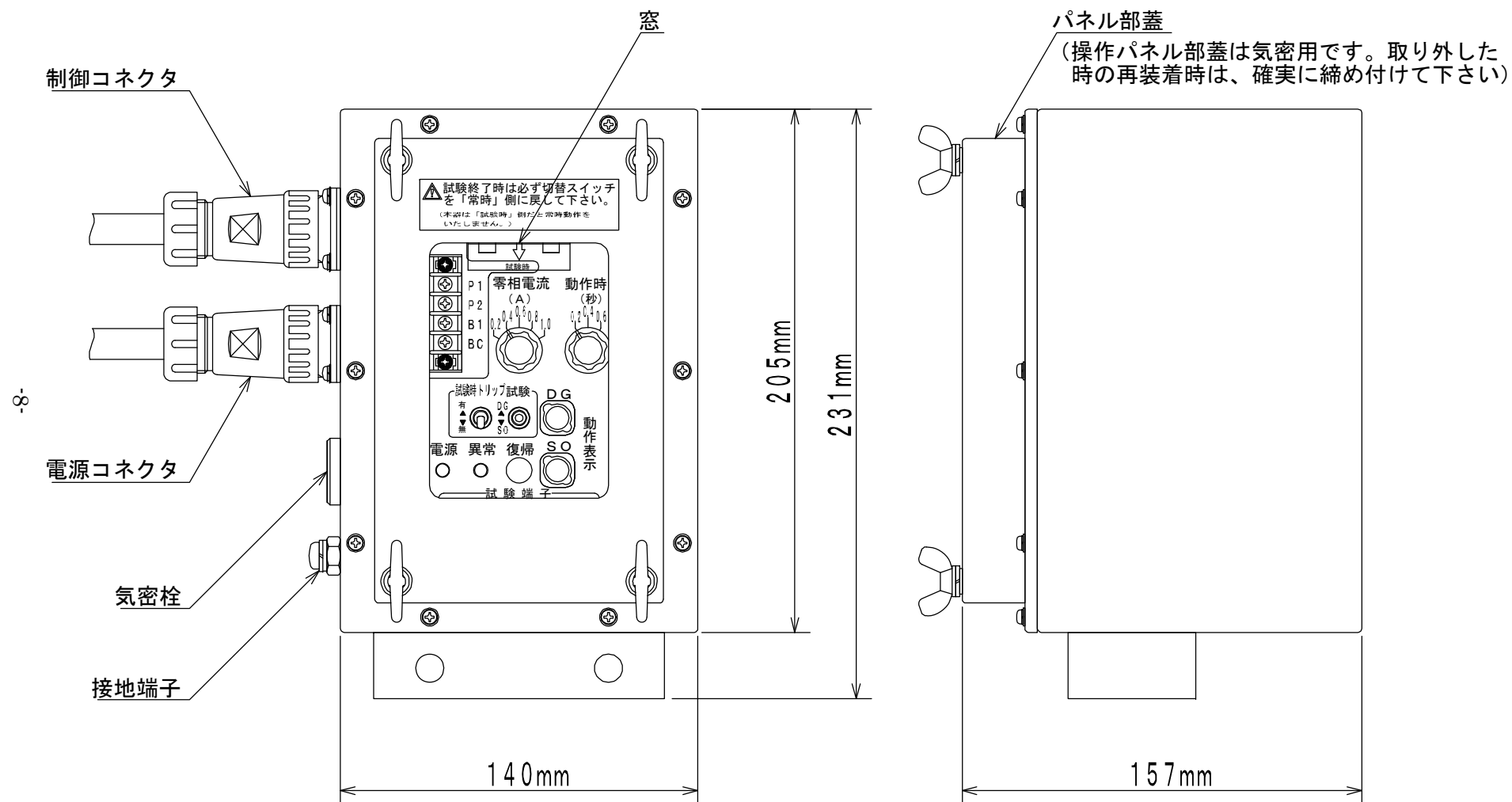
図-3 制御装置外観図（型式 RM634）
