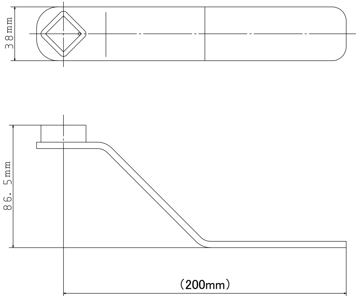
図-2 開閉器操作ハンドル (開閉器を手動で操作する場合に使用します。)
