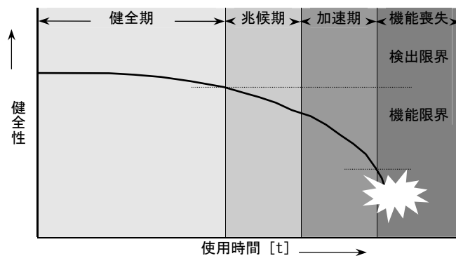
図 14. 劣化故障の進行
