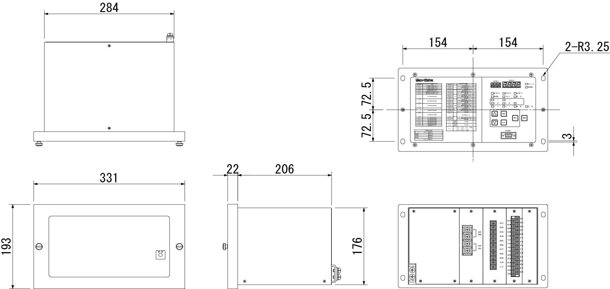
添付資料 1 単独運転検出装置 (QA602) 外観図
