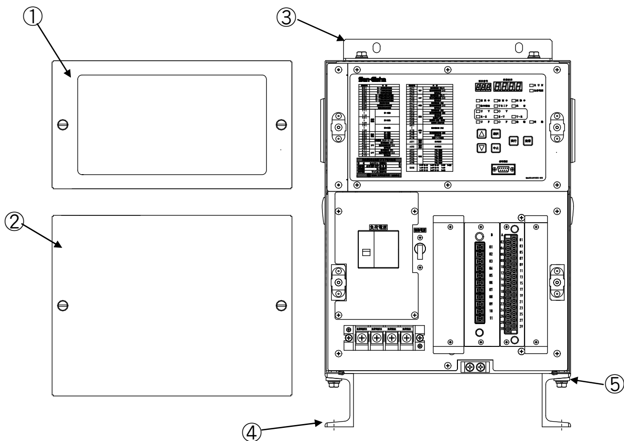
図 III-1 装置（全体）
