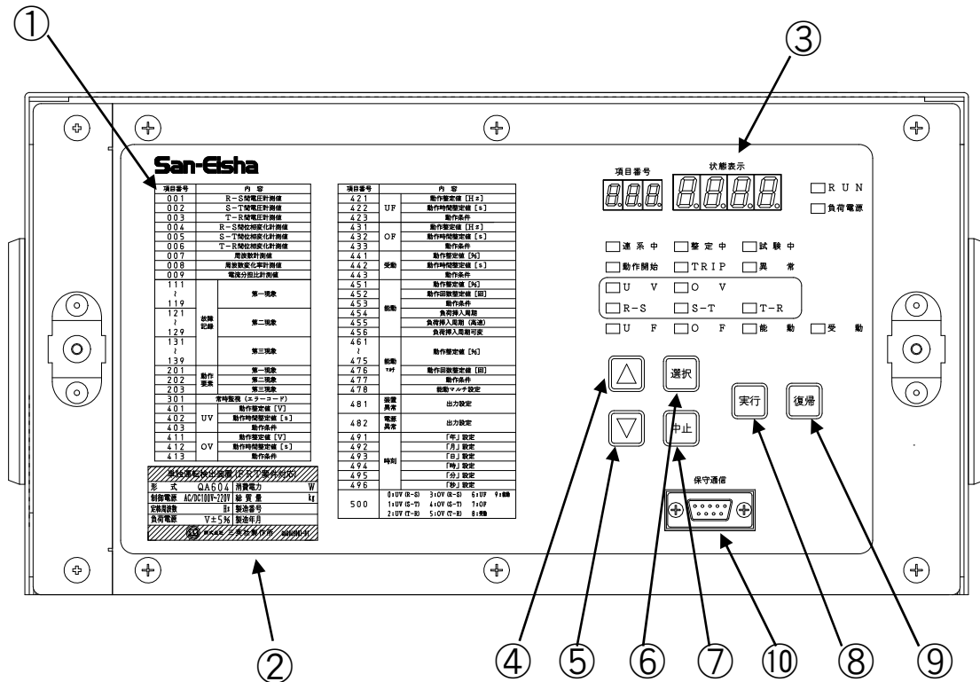
図 III-2 装置（上部）
