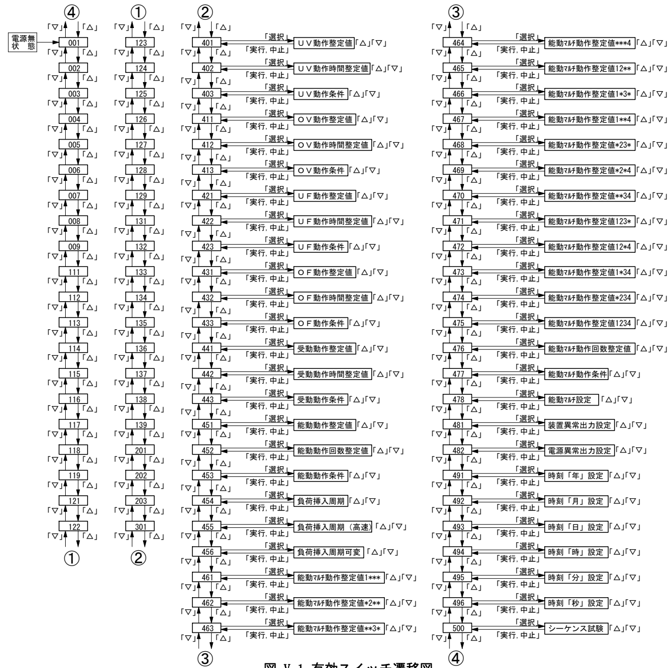
図 V-1 有効スイッチ遷移図
