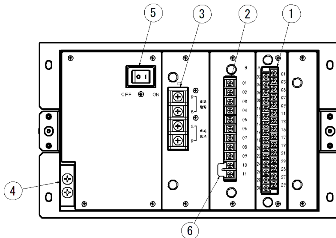
図 III-2 装置（背面）説明一覧表
