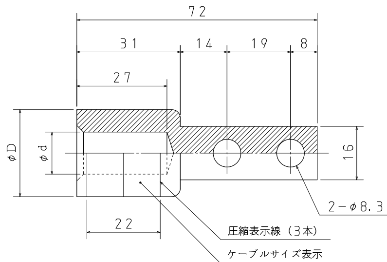
圧縮端子 外観図
