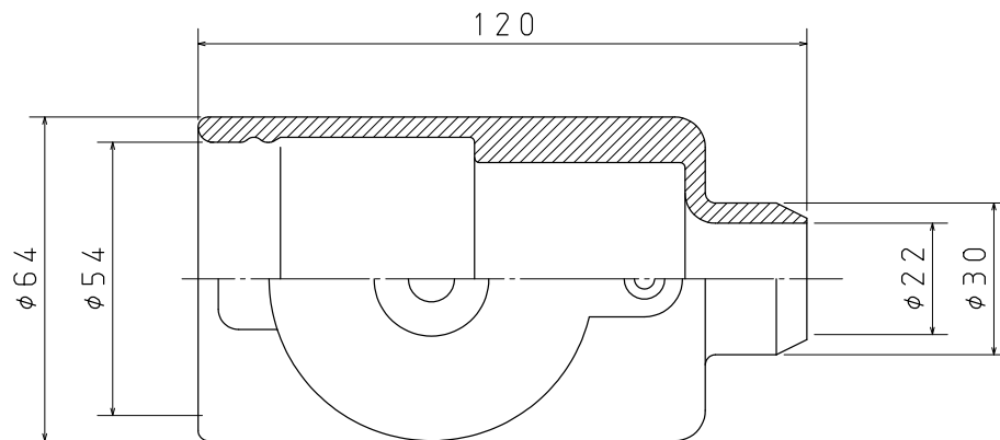
V・UAS90P用端子カバー 外観図
